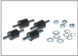
M3 Anti vibration mount. 9g Part No: 1071 M4 Anti vibration mount. 30g Part No: 1072
